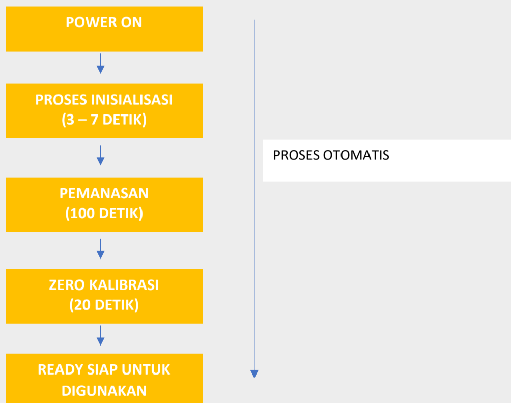
Gambar flow chart proses inisialisasi
