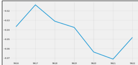
Gambar 17. Grafik Forecasting 7 Hari Parameter Temperatur Kedalaman 30 cm
