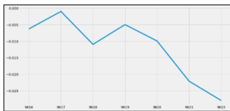
Gambar 19. Grafik Forecasting 7 Hari Parameter Turbidity Kedalaman 30 cm
