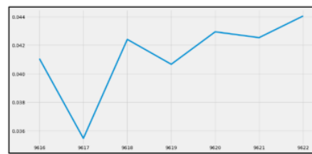
Gambar 20. Grafik Forecasting 7 Hari Parameter Temperatur Kedalaman 60 cm
