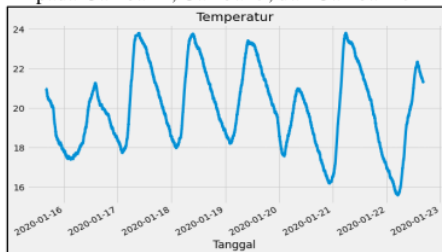
Gambar 2. Plot Parameter Temperatur Kedalaman 30 cm
