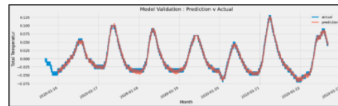
Gambar 15. Grafik Forecasting Parameter Temperatur Kedalaman 60 cm
