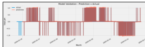
Gambar 14. Grafik Forecasting Parameter Turbidity Kedalaman 30 cm
