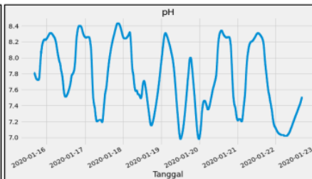
Gambar 3. Plot Parameter pH Kedalaman 30 cm
