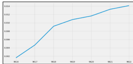
Gambar 21. Grafik Forecasting 7 Hari Parameter Turbidity Kedalaman 60 cm
