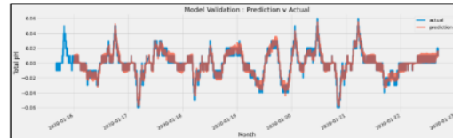
Gambar 13. Grafik Forecasting Parameter pH Kedalaman 30 cm
