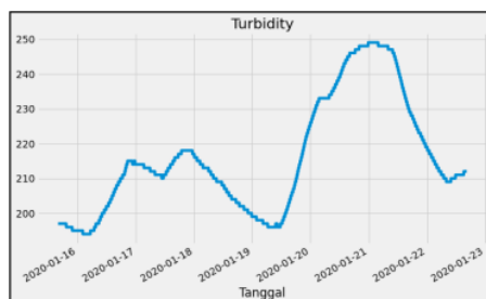
Gambar 4. Plot Parameter Turbidity Kedalaman 30 cm
