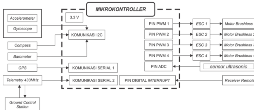
Gambar 4. Arsitektur elektronik quadrotor
