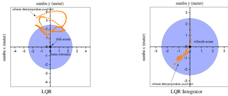
Gambar 8. Hasil pengendalian quadrotor mempertahankan posisi pengujian ke - 4
