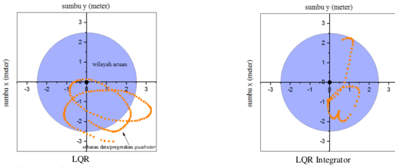
Gambar 7. Hasil pengendalian quadrotor mempertahankan posisi pengujian ke - 3
