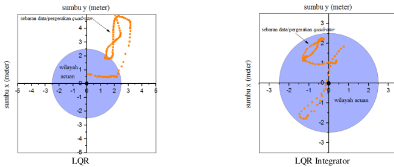
Gambar 9. Hasil pengendalian quadrotor mempertahankan posisi pengujian ke - 5
