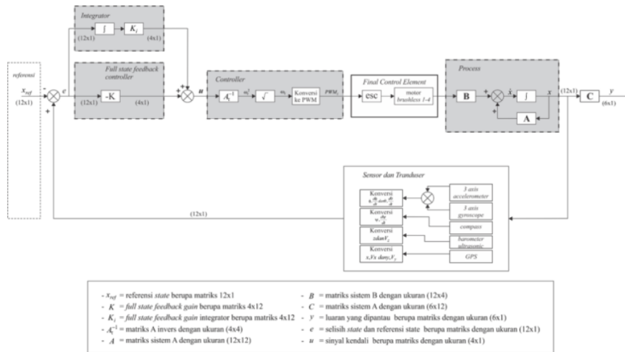
Gambar 2. Diagram blok sistem kendali quadrotor menggunakan metode LQR dan kompensasi Integrator
