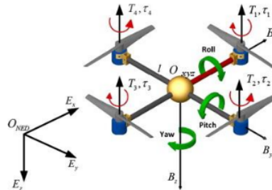
Gambar 1. Quadrotor dengan kerangka acuan NED [8]
