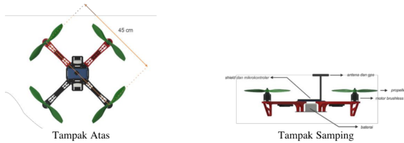
Gambar 3. Desain mekanik quadrotor
