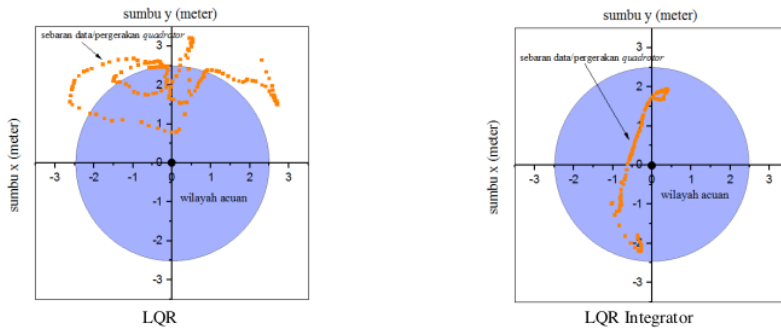
Gambar 6. Hasil pengendalian quadrotor mempertahankan posisi pengujian ke - 2
