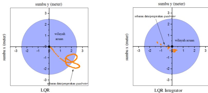
Gambar 5. Hasil pengendalian quadrotor mempertahankan posisi pengujian ke - 1
