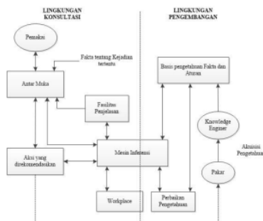
Gambar 2. Struktur Sistem Pakar [3]
