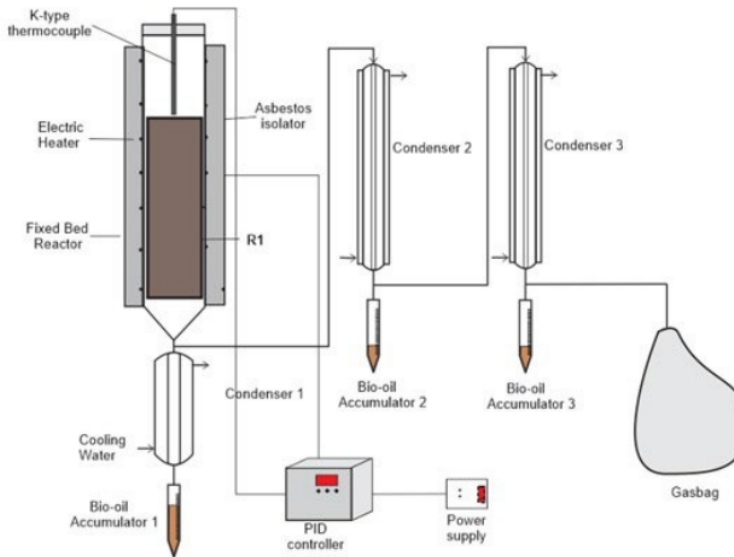
Gambar 1. Unit pirolisis ampas tebu
