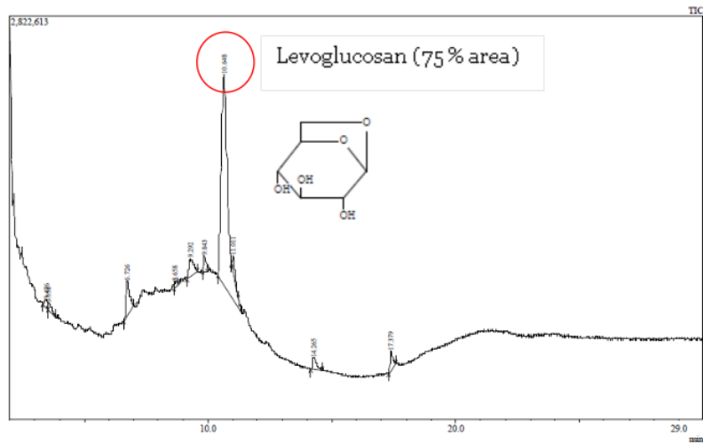
Gambar 5. Hasil GC-MS produk cair pirolisis ampas tebu
