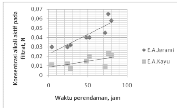
Gambar 2. Konsentrasi alkali aktif filtrat pada berbagai waktu perendaman
