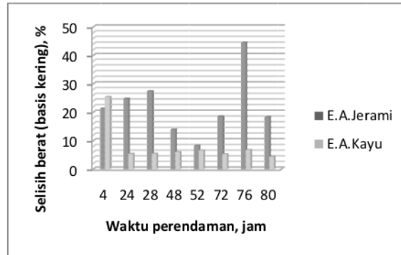
Gambar 1. Pengaruh waktu perendaman dalam ekstrak abu terhadap selisih berat basis kering
