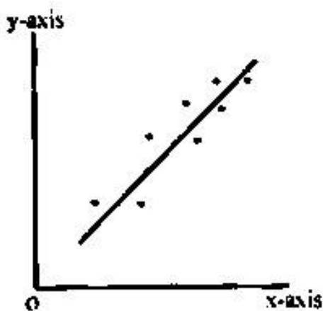
Model Linier
