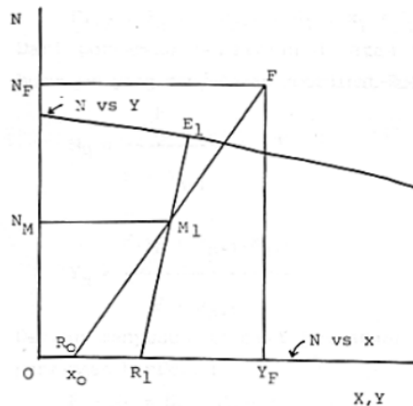
Gambar 3. Grafik ekstraksi untuk sistem bertahap tunggal
