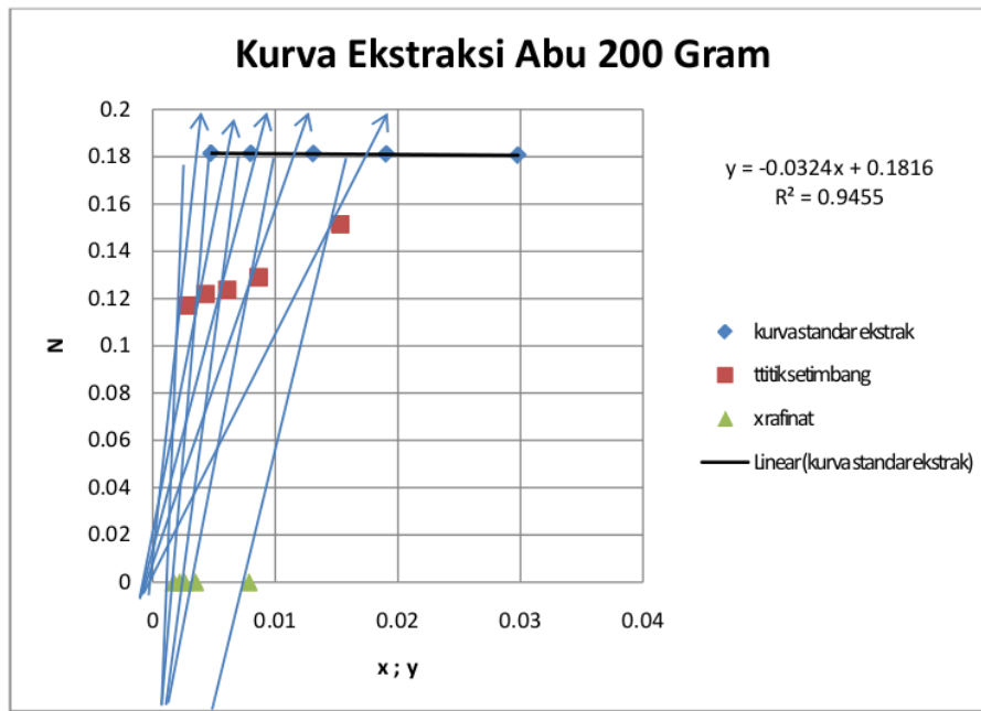
Gambar 4. Grafik rangkaian 5 ekstraksi untuk sistem bertahap tunggal dengan umpan segar berupa abu kayu 200 gram.
