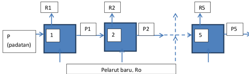
Gambar 1. Sistem bertahap banyak beraliran silang
