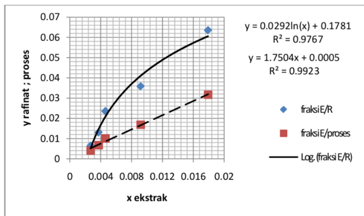
Grafik 3. Hubungan antar fraksi berat pada ekstraksi abu kayu 400 gram.
