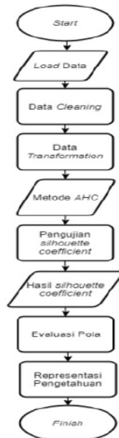
Gambar 1. Metodologi Penelitian
