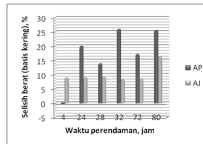
Gambar 1. Pengaruh waktu perendaman terhadap selisih berat basis kering (AP= Ekstrak Abu Kelopak Batang Pisang; AJ=Ekstrak Abu Jerami Padi)
