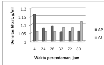
Gambar 3. Densitas filtrat pada berbagai waktu perendaman (AP= Ekstrak Abu Kelopak Batang Pisang; AJ=Ekstrak Abu Jerami Padi)
