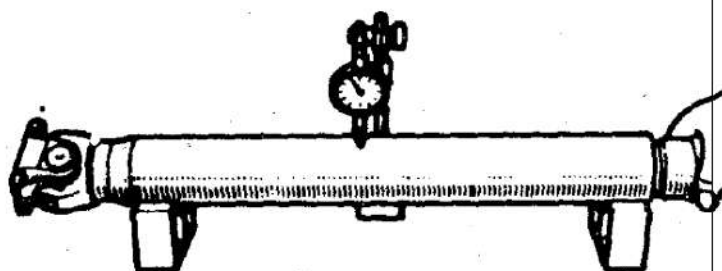
Gb. 26. Memeriksa kebengkokan poros propeller
