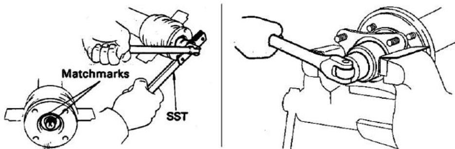
Gb. 16. Melepas mur penahan
