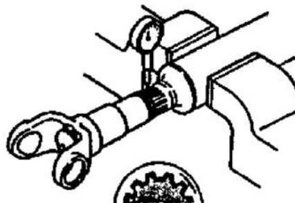
Gb. 24. Mengukur kecocakan alur sleeve
