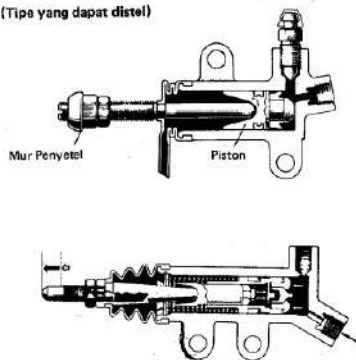
Gb. 16. Release silinder dengan penyetelan
