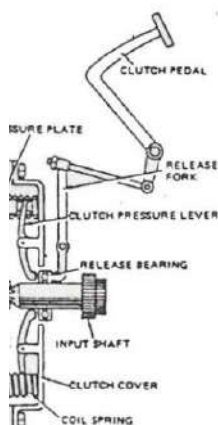
Gb. 1. Mekanisme Mekanik Linkage
