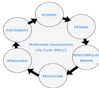
GAMBAR 1. Tahapan MDLC
