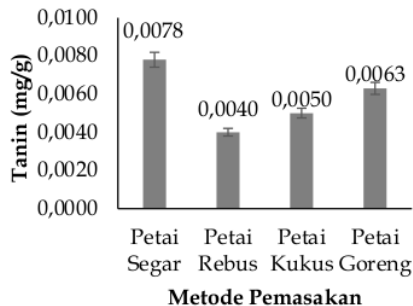
Gambar 2. Perubahan Konsentrasi Antigiizi Tanin Selama Proses Pemasakan
