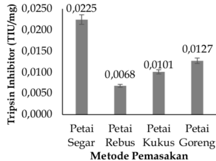
Gambar 3. Perubahan Konsentrasi Antigiizi Tripsin Inhibitor Selama Proses Pemasakan
