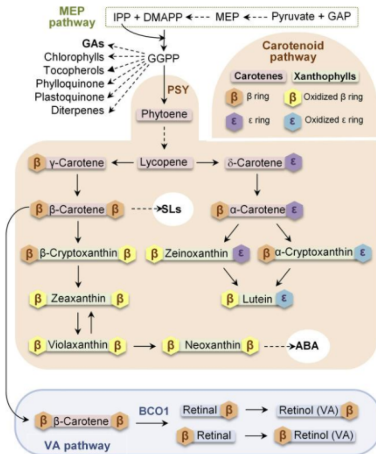
Gambar 5. 9. Biosintesis karotenoid.
