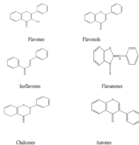
Gambar 5. 2. Penggolongan flavonoid
