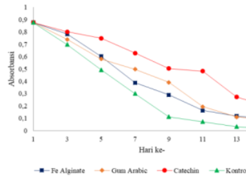
Gambar 2. Grafik Nilai Absorbansi pada Uji Stabilitas Penyimpanan Suhu Ruang
