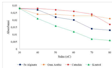
Gambar 3. Grafik Nilai Absorbansi pada Uji Stabilitas Pemanasan
