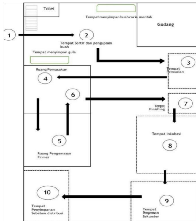
Gambar 1.18 Layout Bangunan Pokok CV. Gemilang Kencana
