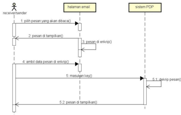
Gambar 6. Sequence diagram baca email dengan proses dekripsi
