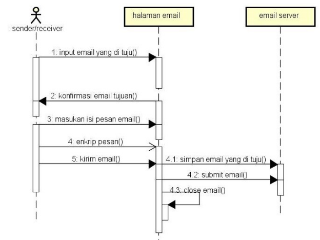
Gambar 5. Sequence diagram kirim email dengan proses enkripsi.
