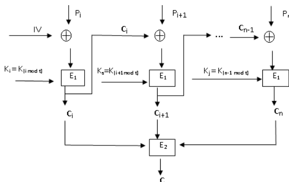
Gambar 1. Skema algoritma CBC termodifikasi (Astuti: 2012)
