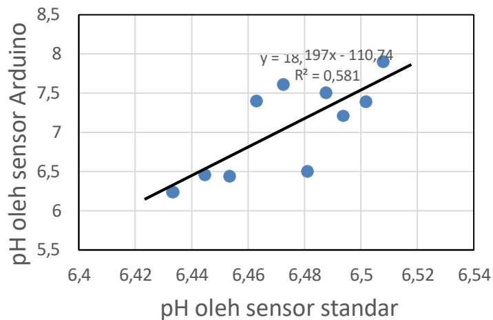
Gambar 21. Kalibrasi sensor pH berbasis arduino dengan sensor pH standar Loggerpro
