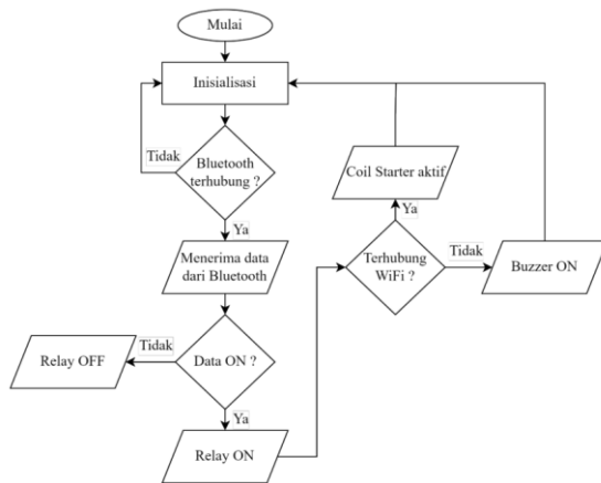
Gambar 5. Flow Chart Perangkat Transmitter
