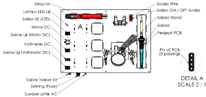
Gambar 6. Desain Dilengkapi Dengan Detail Penunjukan Komponen
