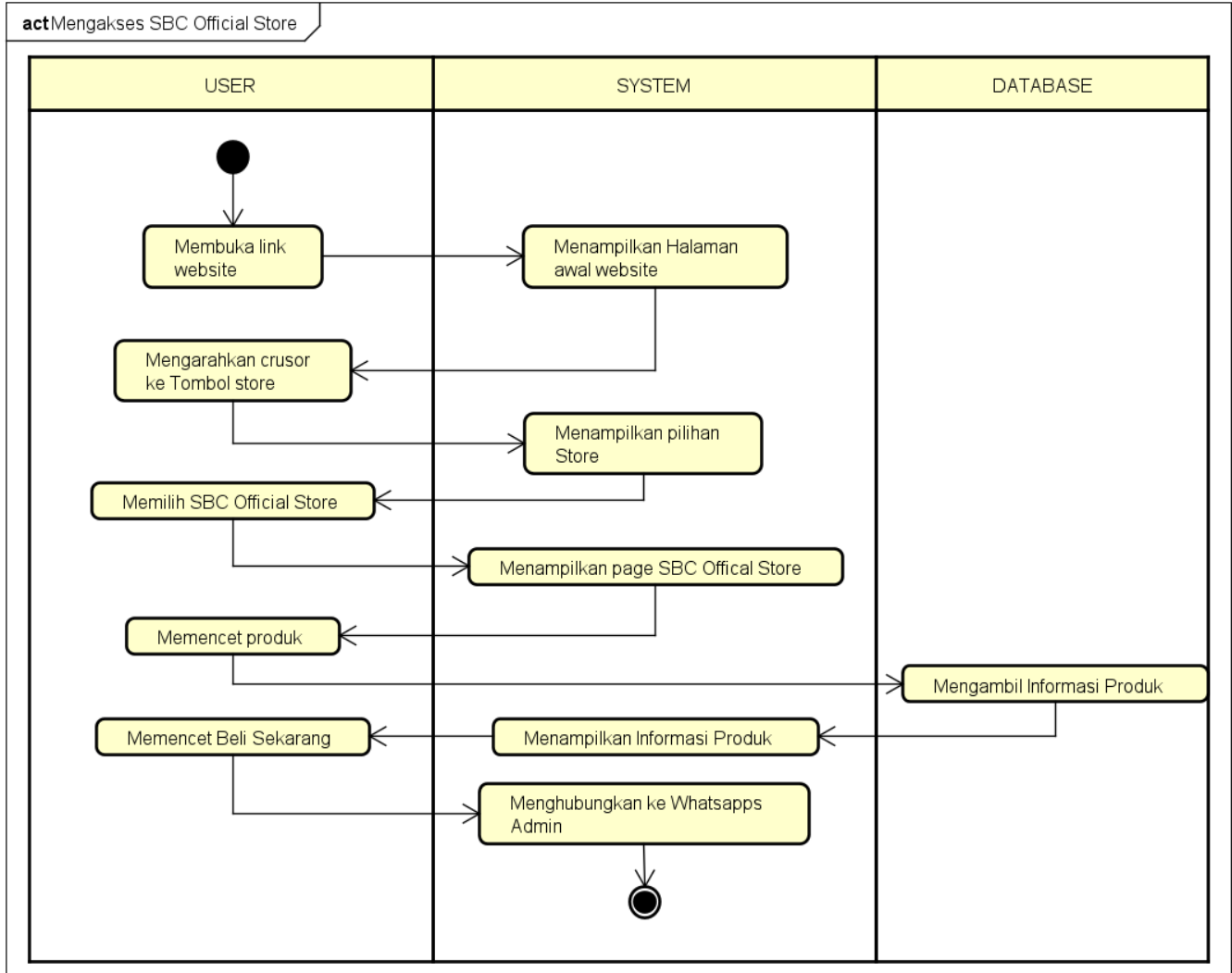
Gambar 4. 14 Activity user tokosaudarasbc mengakses produk SBC Official Store
