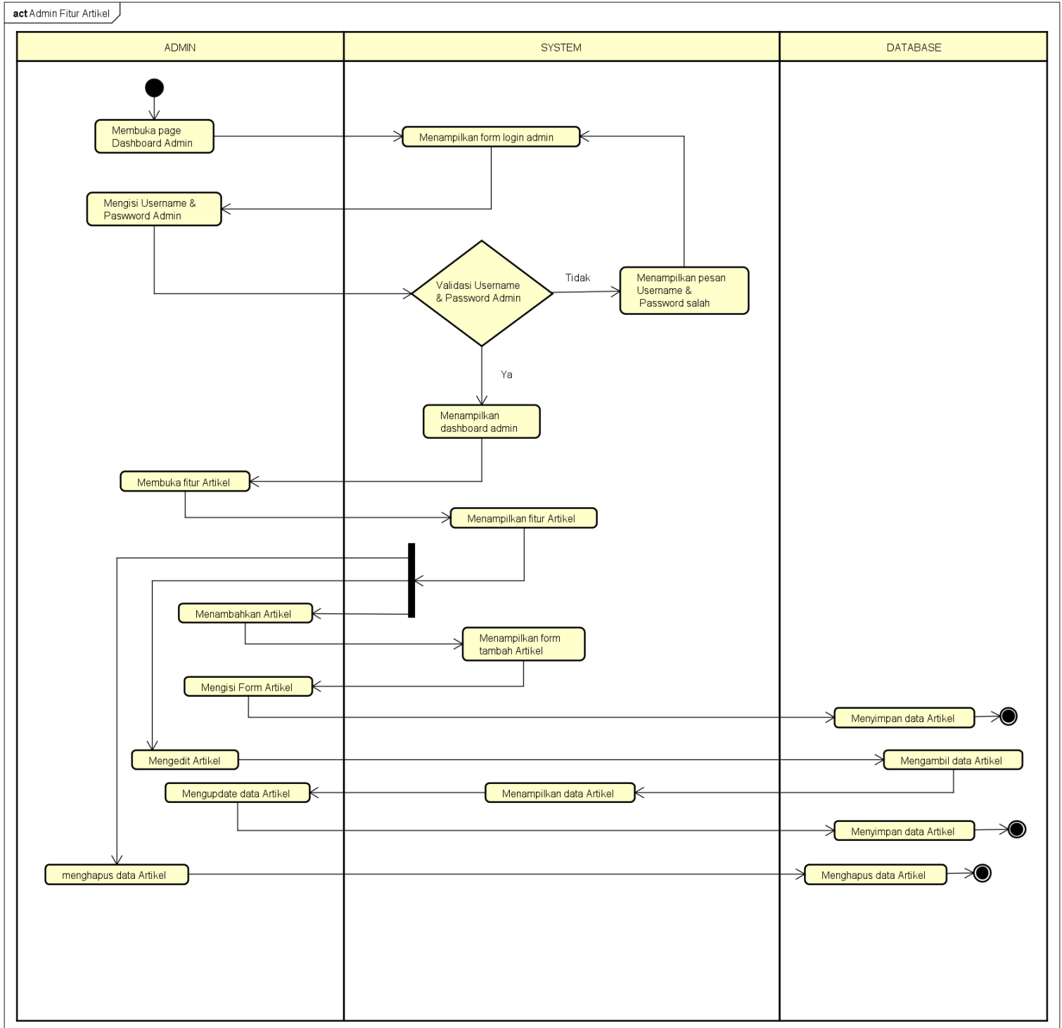
Gambar 4. 6 Activity Admin asaprimaniaga fitur artikel
