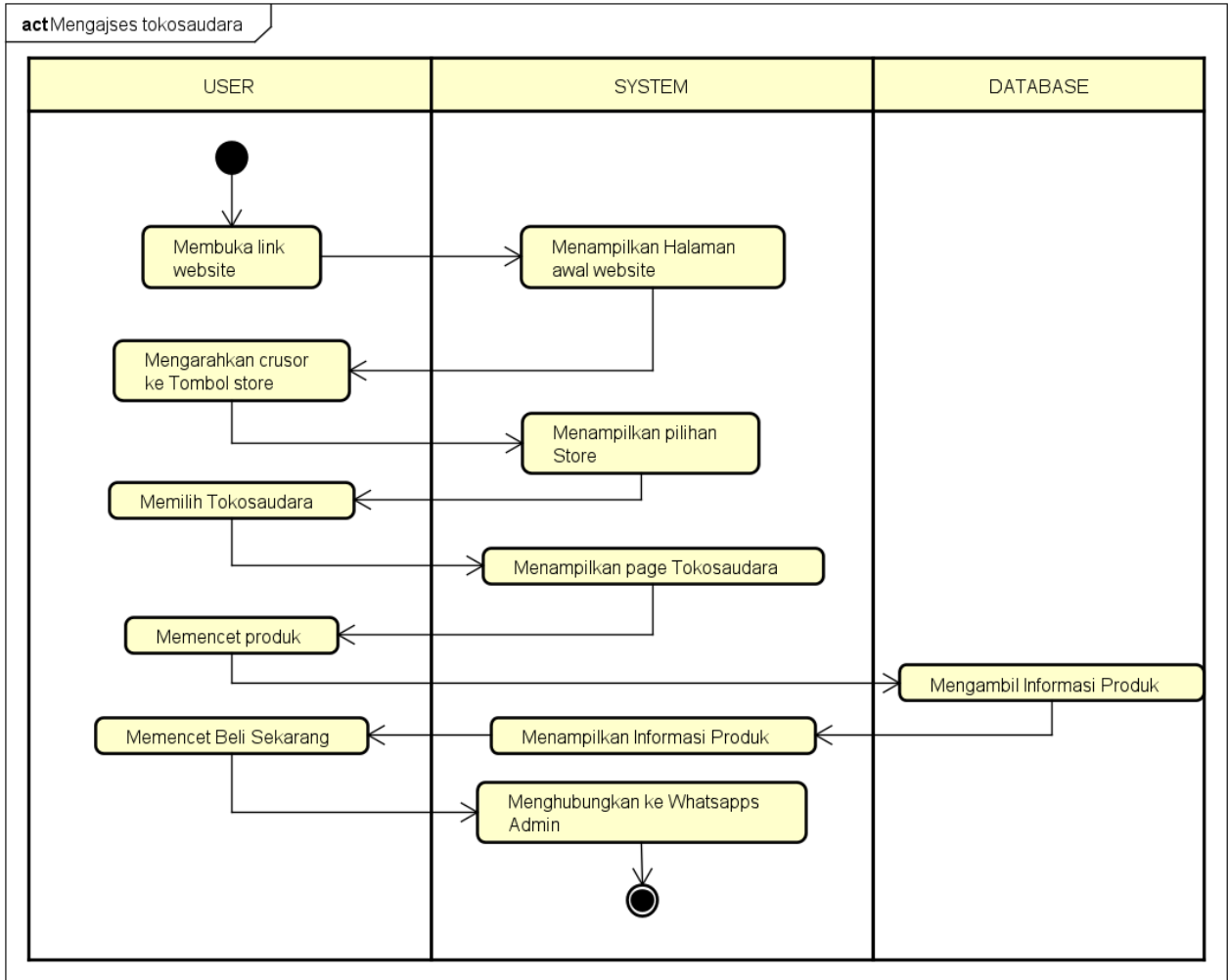
Gambar 4. 13 Activity user tokosaudarasbc mengakses produk toko saudara
