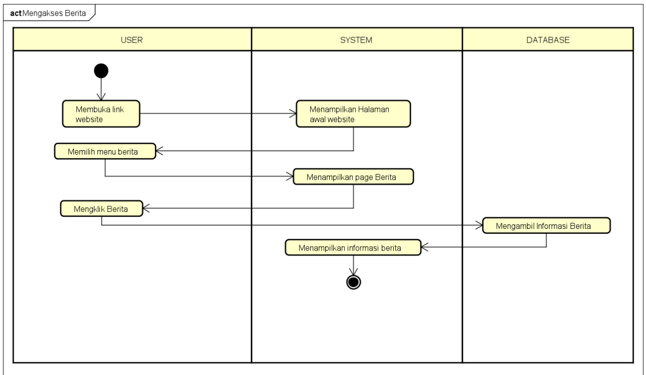
Gambar 4. 12 Activity user tokosaudara sbc mengakses berita
