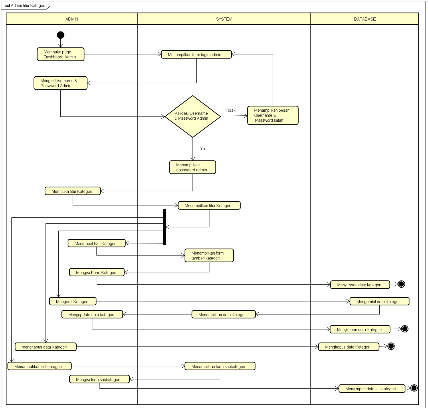
Gambar 4. 11 Activity Admin asaprimaniaga fitur kategori
