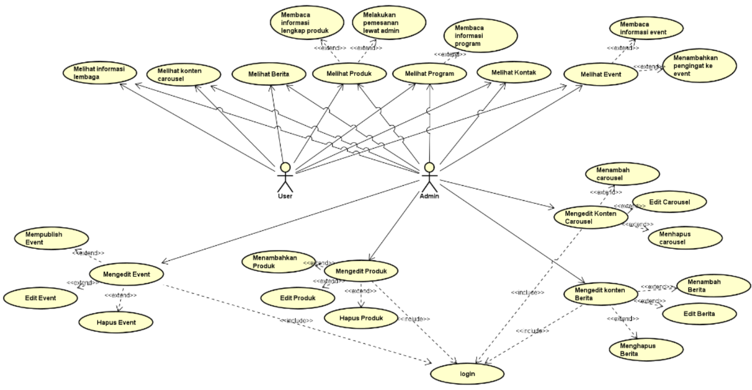
Gambar 4. 22 Use Case diagram tokosaudarasbc.com
