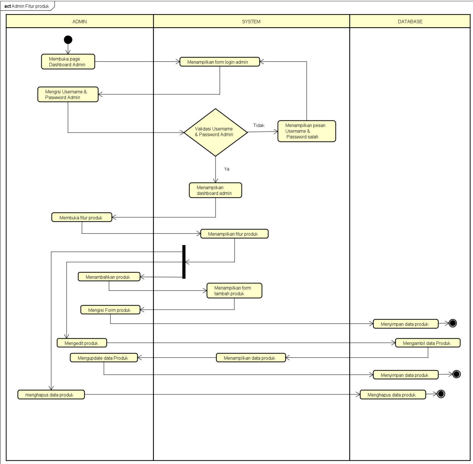
Gambar 4. 8 Activity Admin asaprimaniaga fitur produk
