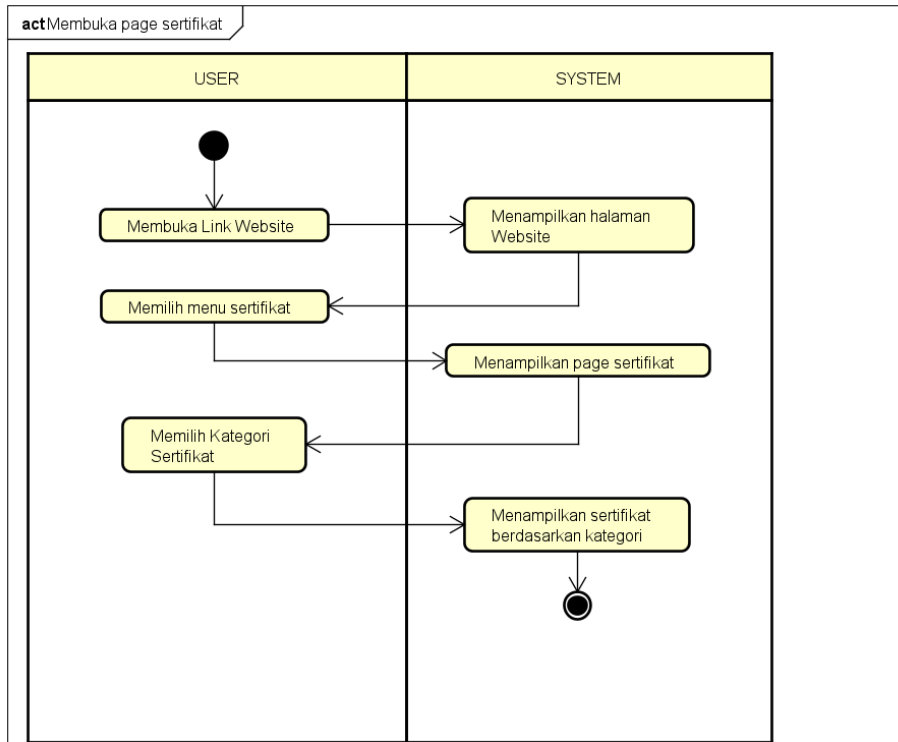
Gambar 4. 4 Activity User asaprimaniaga membuka page sertifikat
