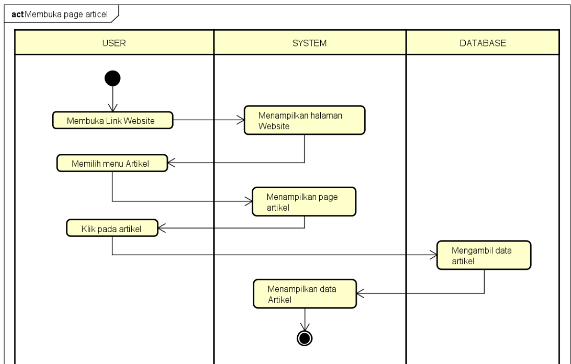
Gambar 4. 1 Activity Diagram asaprimaniaga membuka page artikel
