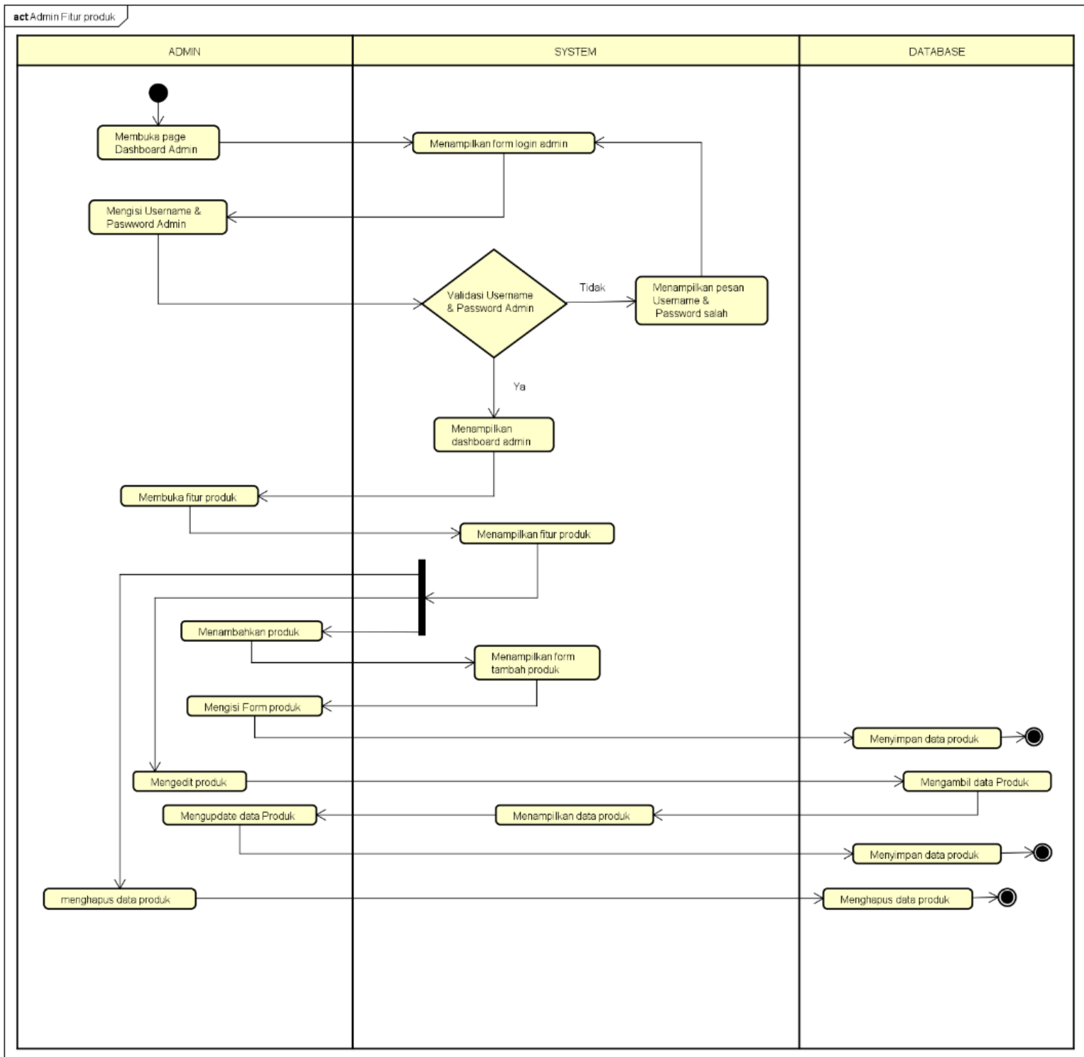
Gambar 4. 17 Activity diagram admin tokosaudara sbc fitur produk
