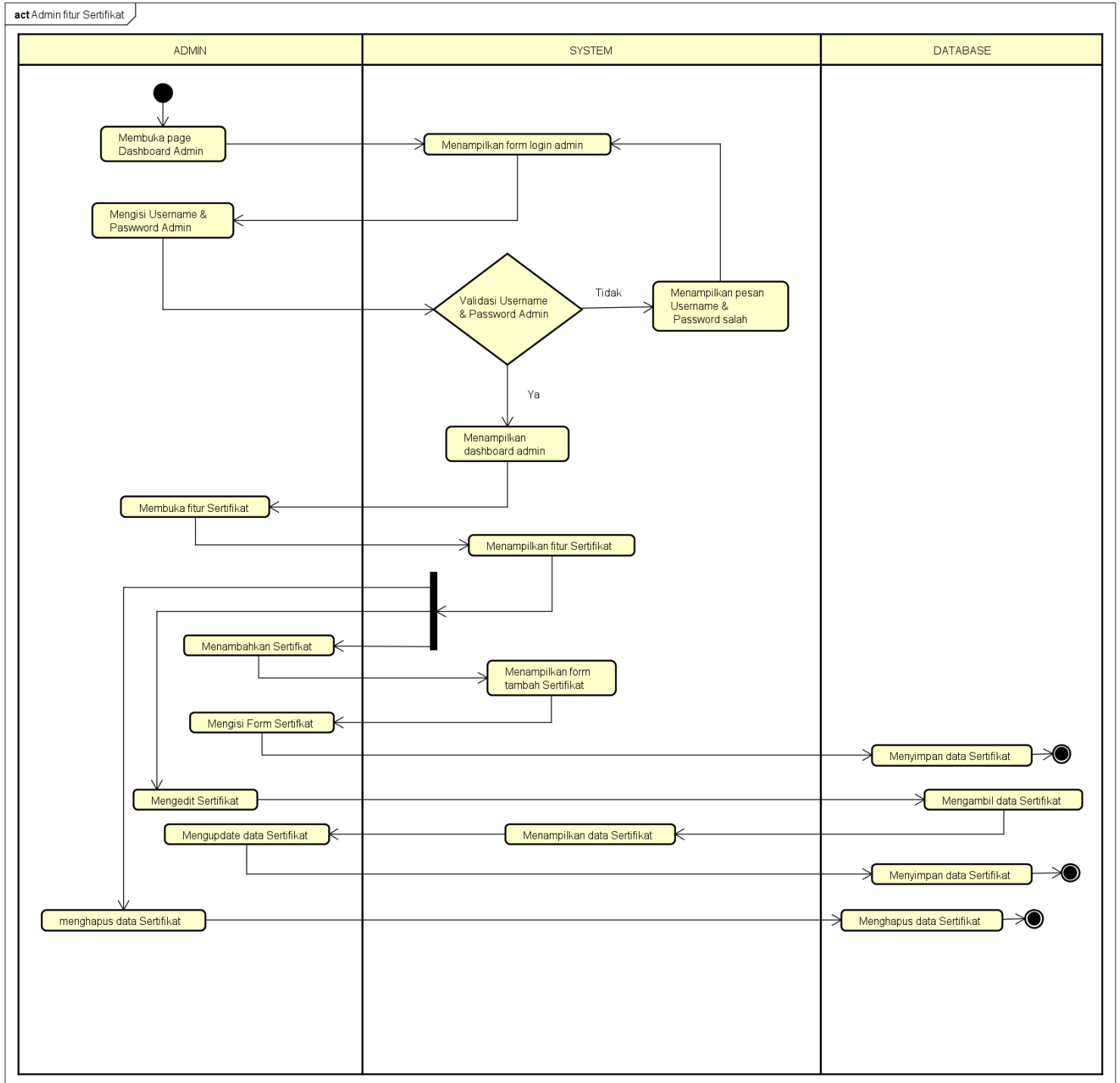
Gambar 4. 10 Activity Admin asaprimaniaga fitur Sertifikat
