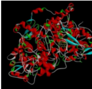
Gambar 5. Ligan dan reseptor hasil docking
