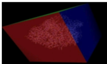
Gambar 3. Reseptor yang sudah di preparasi
