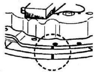
Gb. 14. Memasang unit rumah kopling
