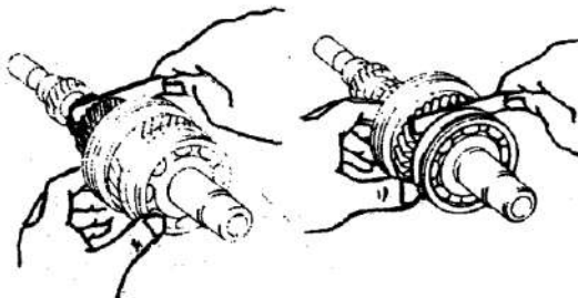
Gb. 3. Pengukuran celah antar gigi
