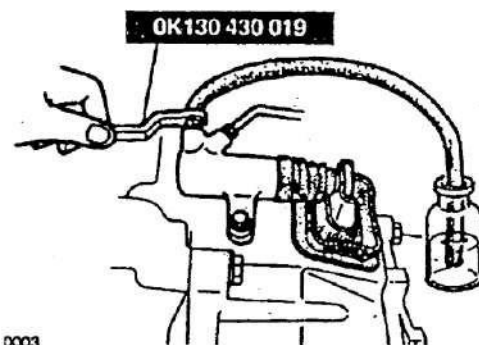
Gb. 22. Mengeluarkan udara dari dalam sistem melalui release silinder
