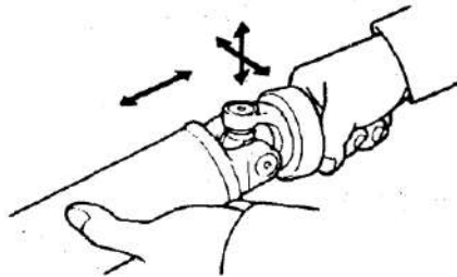
Gb. 25. Memeriksa kekocakan spider
