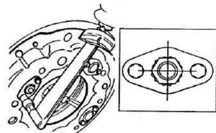
Gb. 16. Pengencangan mur penahan tuas penekan
