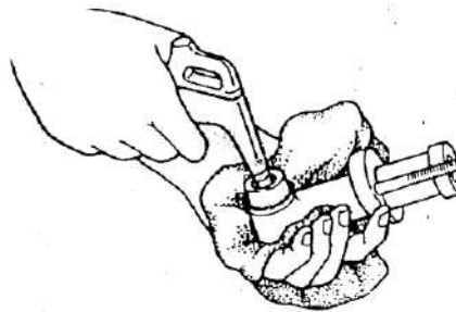
Gb. 9. Mengeluarkan piston unit dengan kompresor
