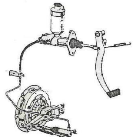
Gb. 3. Mekanisme Hidrolik
