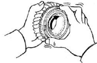
Pemeriksaan hubungan antara roda gigi dan synchronizerring
