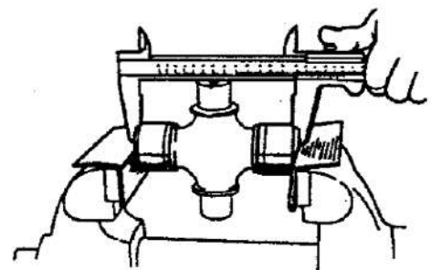
Gb. 28. Memeriksa panjang spider
