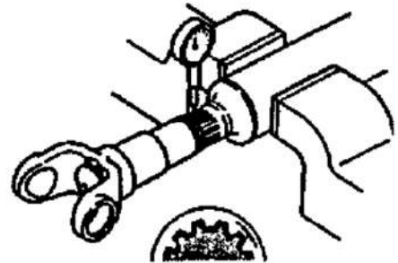
Gb. 24. Mengukur kekocakan alur sleeve
