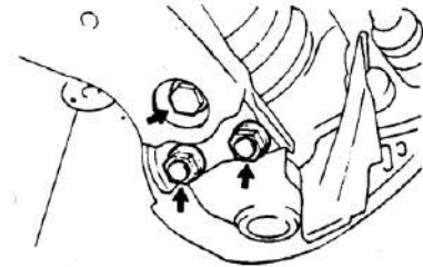
Gb. 6. Melepas steering knuckle dari lower arm
