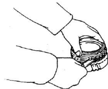
Gb. 5. Pengukuran celah antara gigi dan synchronizerring
