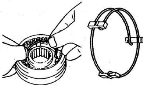
Gb. 9. Pemasangan unit synchromesh
