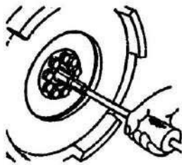
Gb. 13. Melepas pilot bearing (Jika akan diganti)
