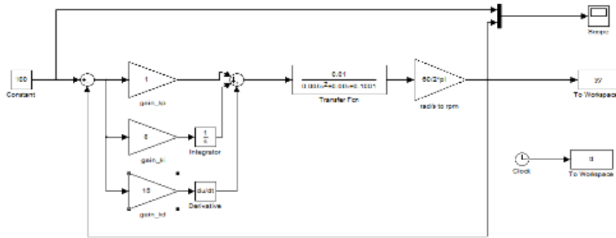
Gambar 5. Plant motor DC pada matlab.
