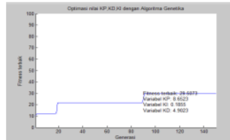
Gambar 17. Hasil simulasi jumlah generasi 150.
