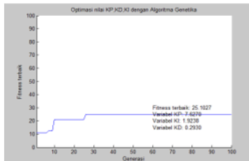
Gambar 8. Hasil simulasi Pmutasi 0,8.
