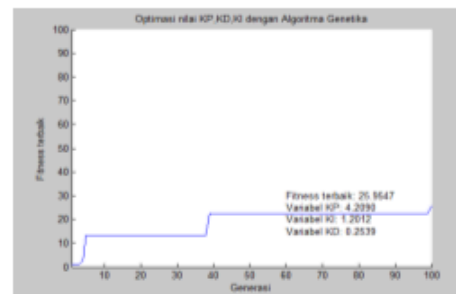
Gambar 13. Hasil simulasi Psilang 0,4.
