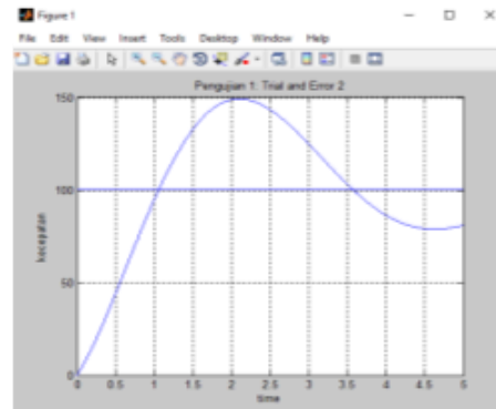
Gambar 7. Grafik data nomor 2 pengujian trial and error .
