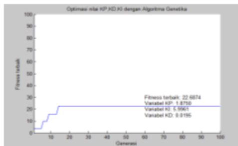
Gambar 12. Hasil simulasi Psilang 0,2.
