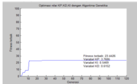
Gambar 16. Hasil simulasi jumlah generasi 120.
