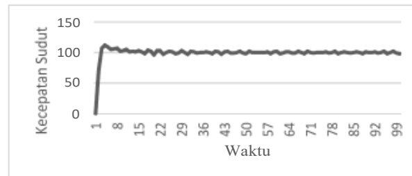
Gambar 23. Grafik metode GA Pmutasi 0,8 pada pengujian hardware .
