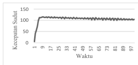
Gambar 28. Grafik metode GA jumlah gen 150 pada pengujian hardware .
