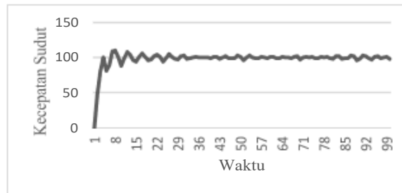
Gambar 25. Grafik metode GA Psilang 0,2 pada pengujian hardware .
