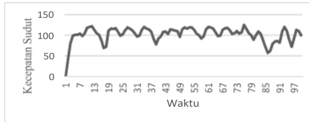
Gambar 21. Grafik metode trial and error 1 pada pengujian hardware .
