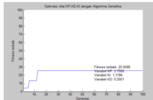
Gambar 9. Hasil simulasi Pmutasi 1.
