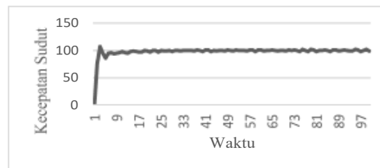
Gambar 27. Grafik metode GA jumlah gen 120 pada pengujian hardware .
