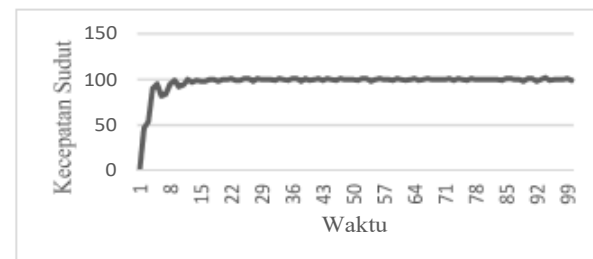
Gambar 24. Grafik metode GA Pmutasi 1 pada pengujian hardware .
