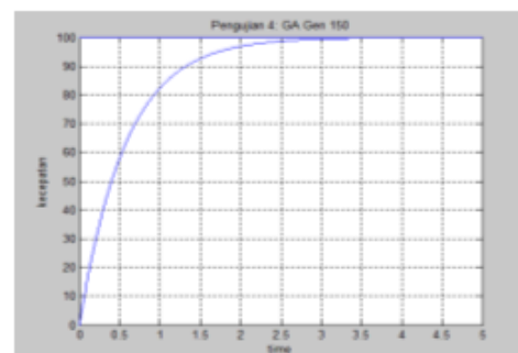
Gambar 19. Grafik hasil simulasi jumlah generasi 150.
