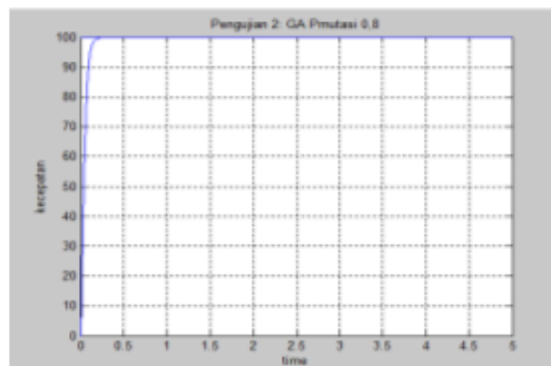
Gambar 10. Grafik hasil simulasi Pmutasi 0,8.
