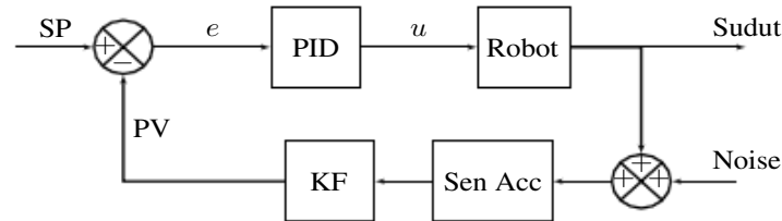
Gambar 2. Diagram Blok Kendali Sistem Kendali Kalang Tertutup
