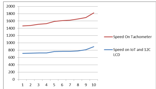
Fig. 7. Grafik pengujian data dalam kondisi kecepatan 50%
