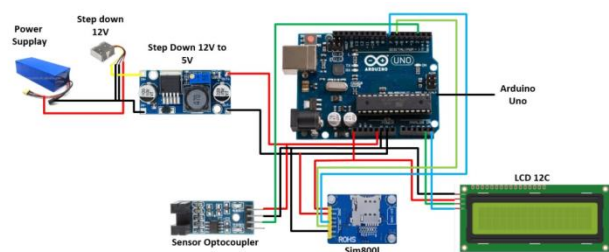
Fig. 3. Wiring diagram
