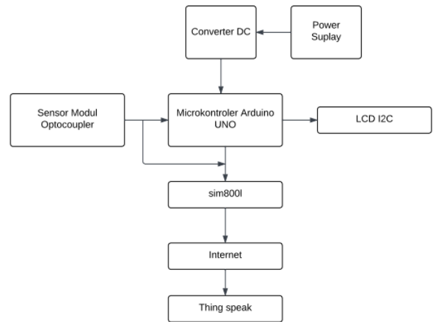
Fig. 2. Blok Diagram
