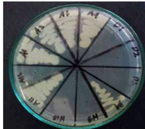
Gambar 2. Hasil pengamatan KBM ekstrak metanol termas terhadap B. subtilis . Tampak pada gambar ekstrak metanol daun (A1, A2, A3), ekstrak metanol batang (D1, D2, D3). kontrol negatif (A11), kontrol media (A12), kontrol positif (H9, H10).
