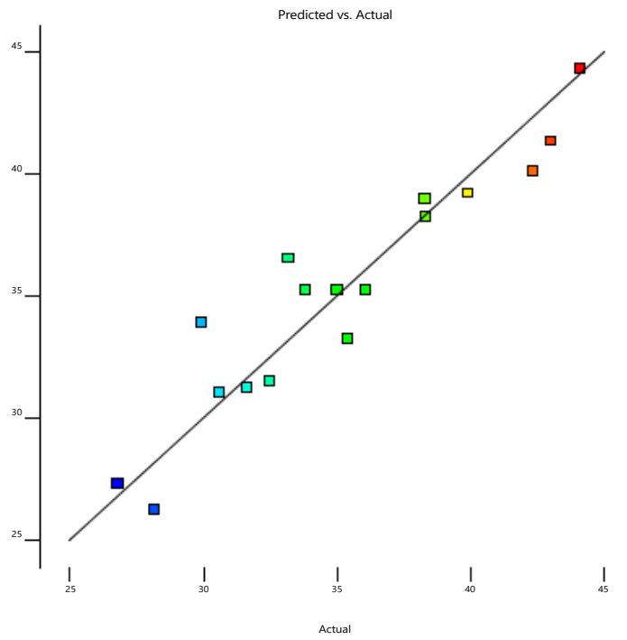
Figure 5. Estimated vs. Actual Values.
