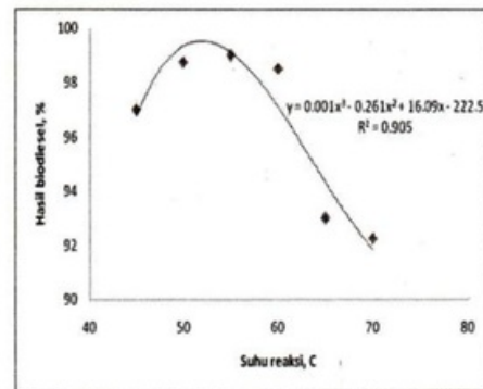
Gambar 1. Grafik Hubungan antara suhu reaksi dan hasil biodiesel
