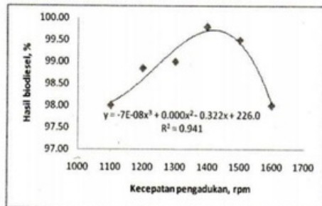
Gambar 2. Grafik Hubungan Antar Kecepatan pengadukan dan Hasil Biodiesel
