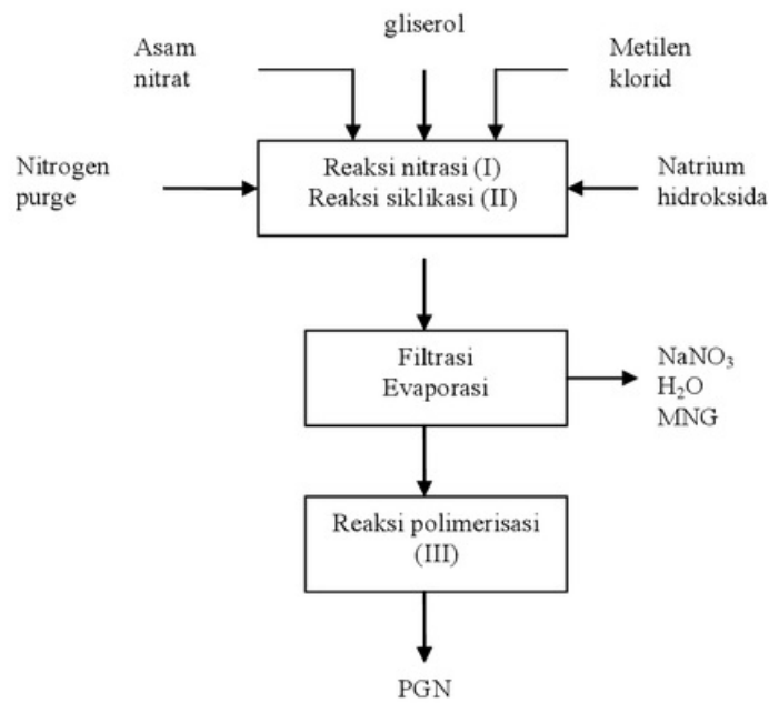
Gambar 1. Proses Pembuatan PGN secara Batch
