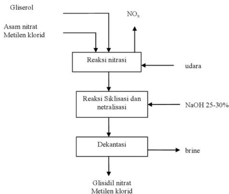
Gambar 2. Proses Pembuatan PGN secara kontinyu (Cara I)
