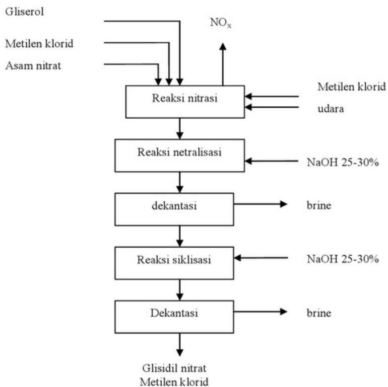
Gambar 3. Proses Pembuatan PGN secara kontinyu (Cara II)
