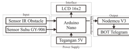
Gambar 2. Diagram blok sistem alat pengukur suhu
