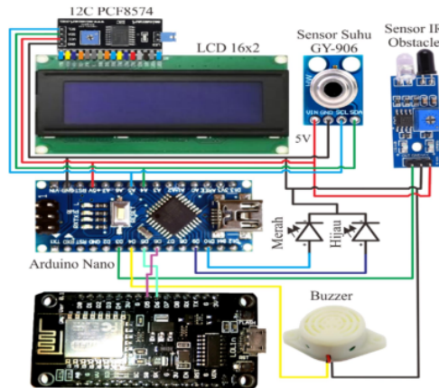
Gambar 3. Wiring sistem alat pengukur suhu
