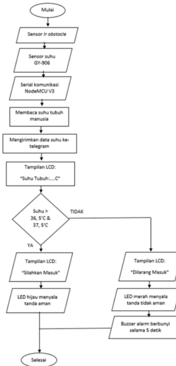
Gambar 5. Rangkaian flowchart sistem
