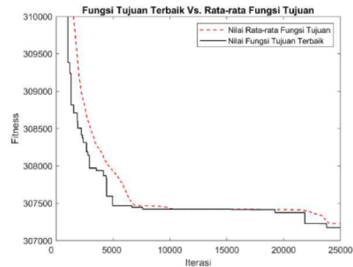
Gambar 3. Grafik Nilai Fungsi Tujuan Vs. Nilai Rata-rata Fungsi Tujuan GA ketika dijalankan ke-4
