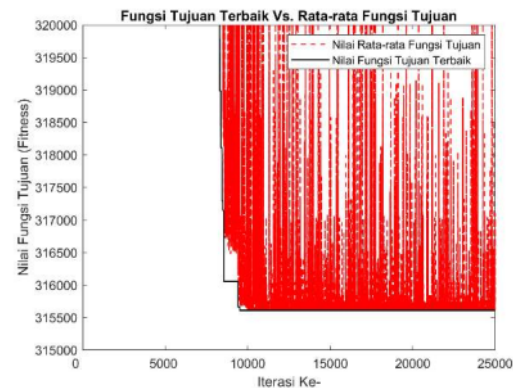
Gambar 4. Grafik Nilai Fungsi Tujuan Vs. Nilai Rata-rata Fungsi Tujuan PSO dijalankan ke-7
