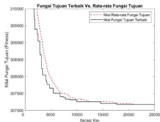
Gambar 2. Grafik Nilai Fungsi Tujuan Vs. Nilai Rata-rata Fungsi Tujuan GA ketika dijalankan ke-3
