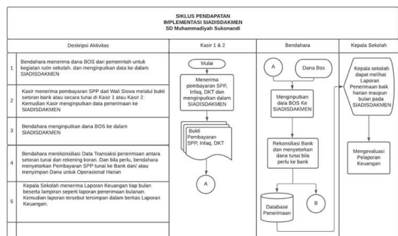
Gambar 2. Flowchart Siklus Pendapatan Sesudah adanya SIADISDAKSMEN
