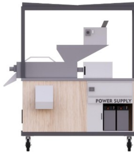
Gambar 1 : Tampak Depan
