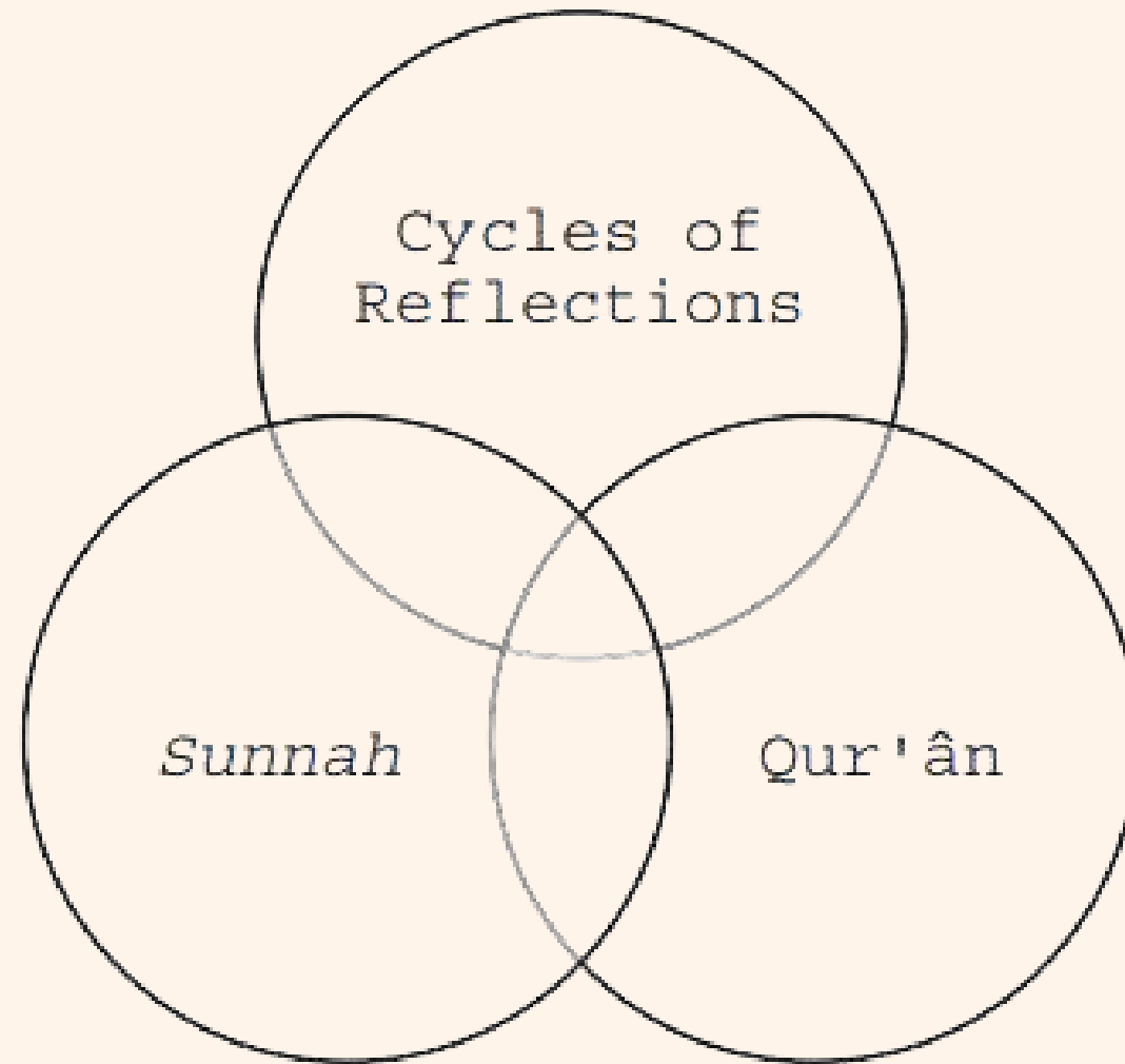
Siklus Refleksi
