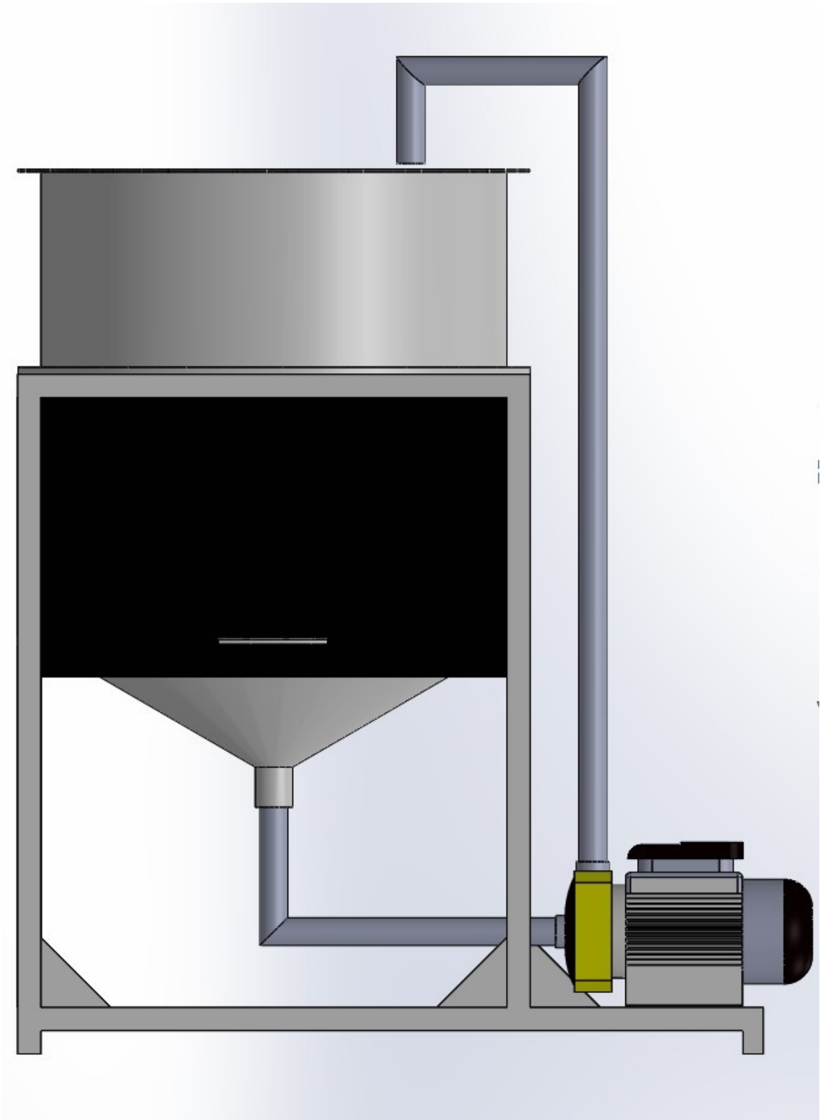
Gambar 2 - Tampak Depan
