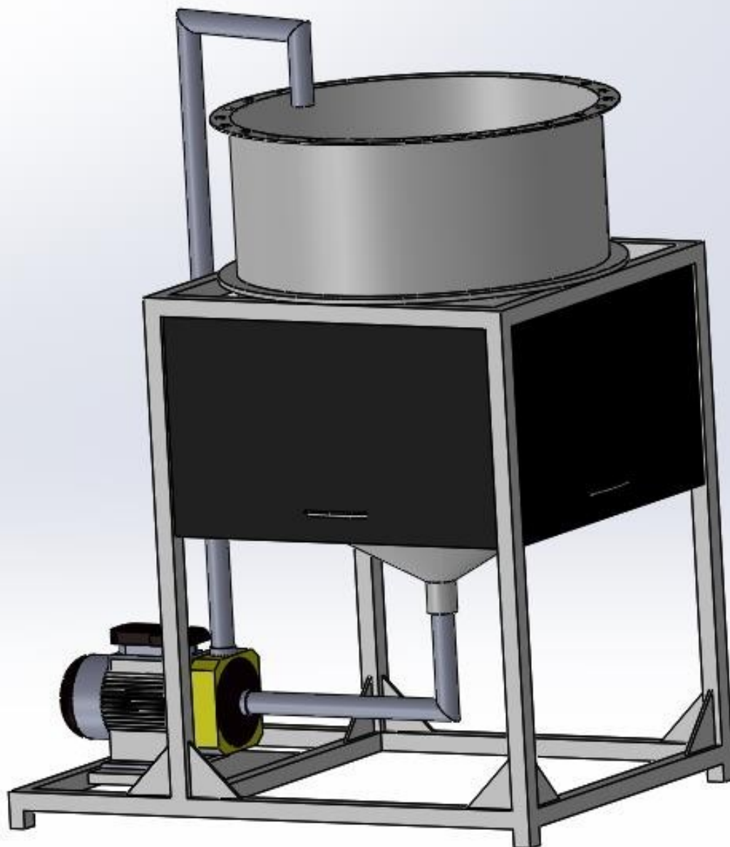
Gambar 1 - Tampak Perspektif
