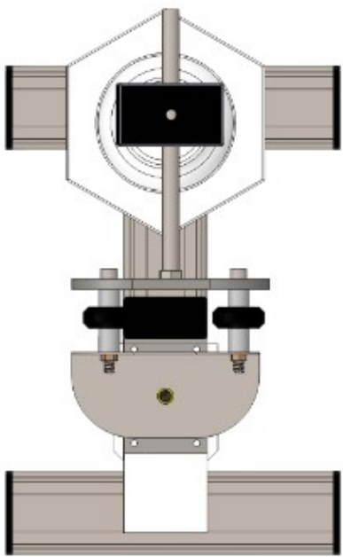
Gambar 5 : Tampak Atas
