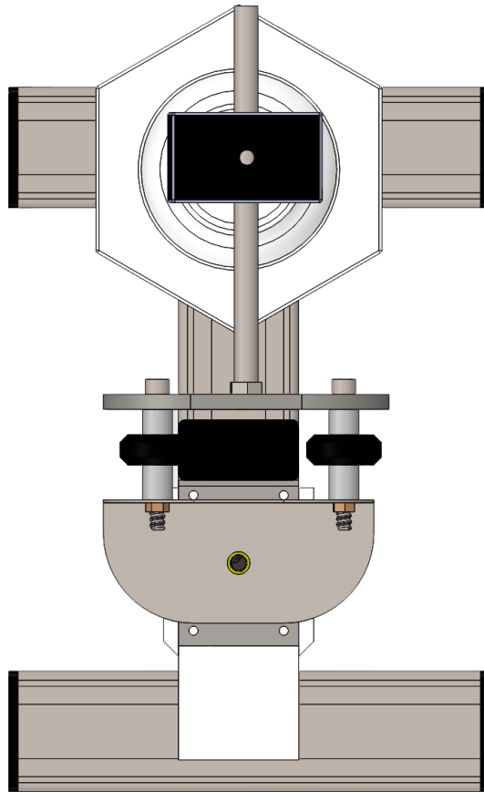
Gambar 5 : Tampak Atas
