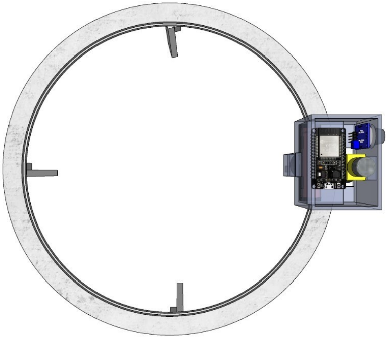
Gambar 6 - Tampak Atas
