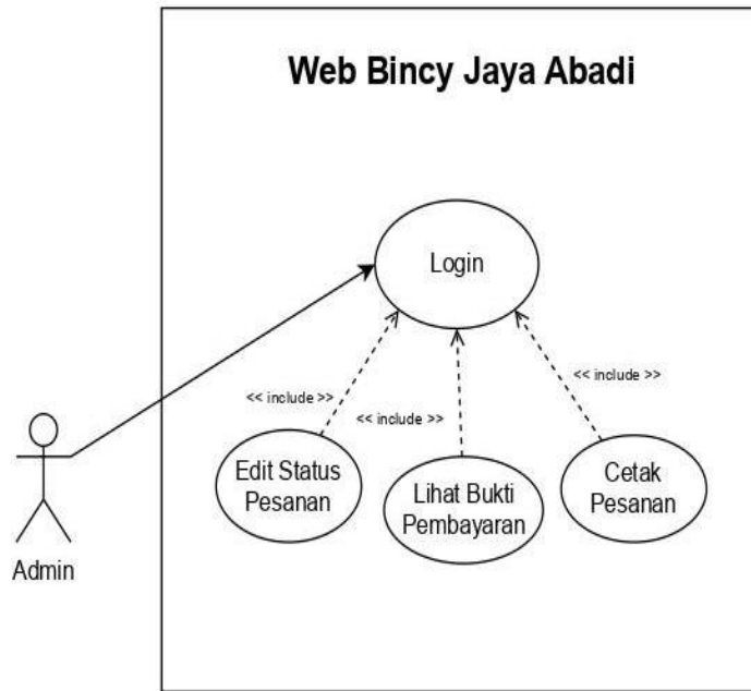
Gambar 3. 14 Use case Admin Pesanan
