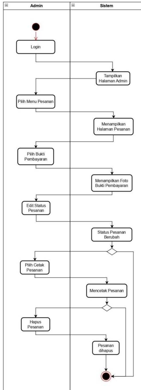
Gambar 3. 10 Aktivitas Login Admin Pesanan
