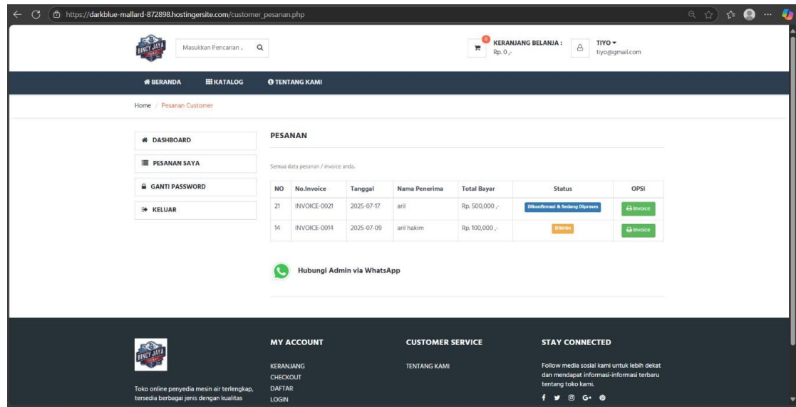
Gambar 3. 36 Halaman Pesanan
