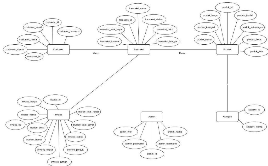
Gambar 3. 19 ERD
