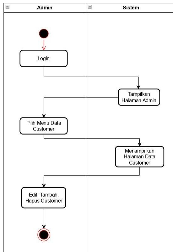
Gambar 3. 6 Aktivitas Login AdminData Costumer
