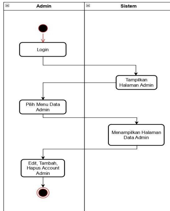
Gambar 3. 5 Aktivitas Login Admin Akun
