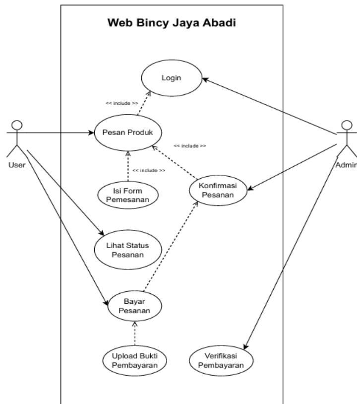
Gambar 3. 11 Use Case Pemesanan
