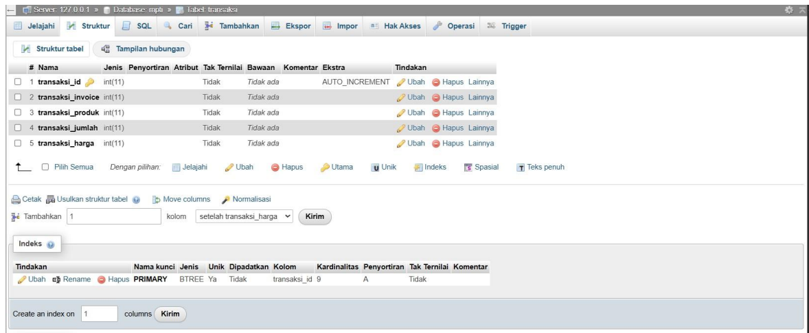
Gambar 3. 25 Tabel Transaksi
