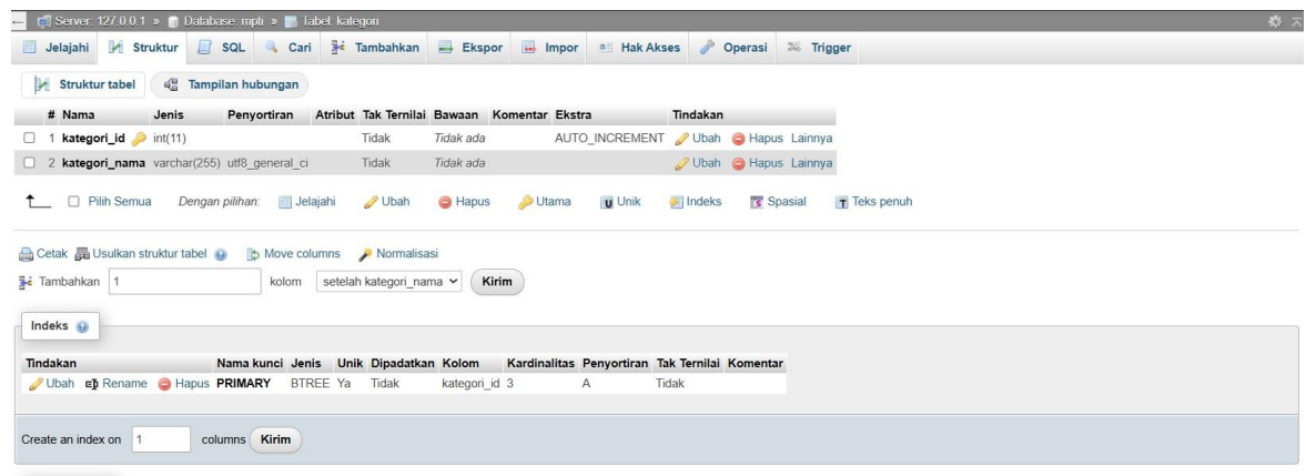
Gambar 3. 23 Tabel kategori
