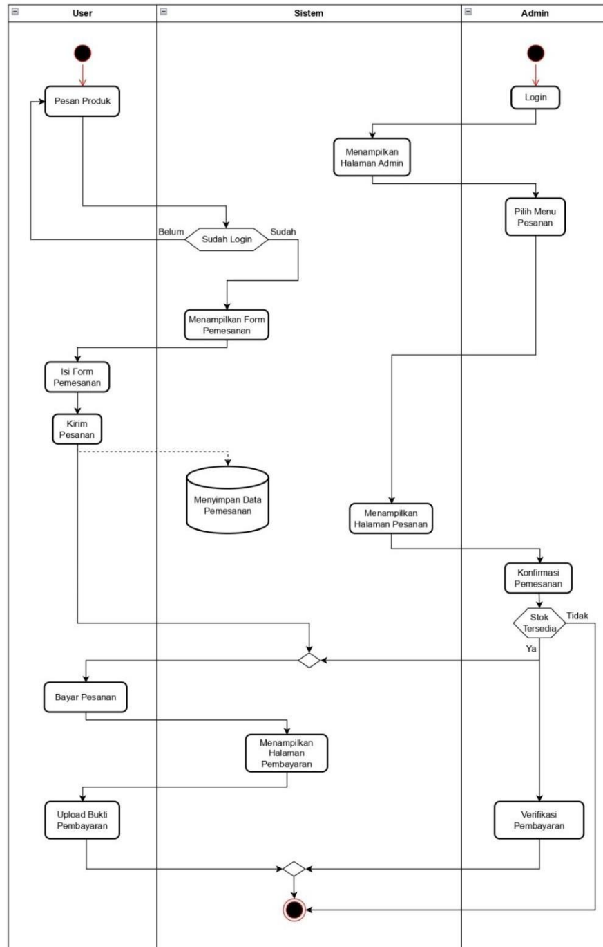
Gambar 3. 3 Aktivitas Pemesanan
