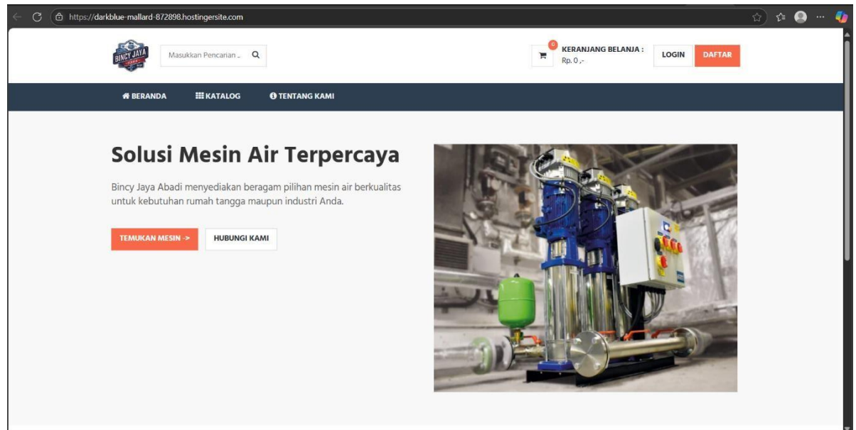
Gambar 3. 30 Halaman Beranda
