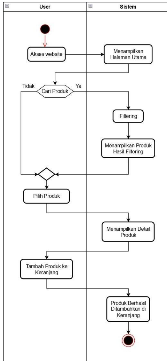
Gambar 3. 4 Aktivitas User melakukan Pencarian Produk
