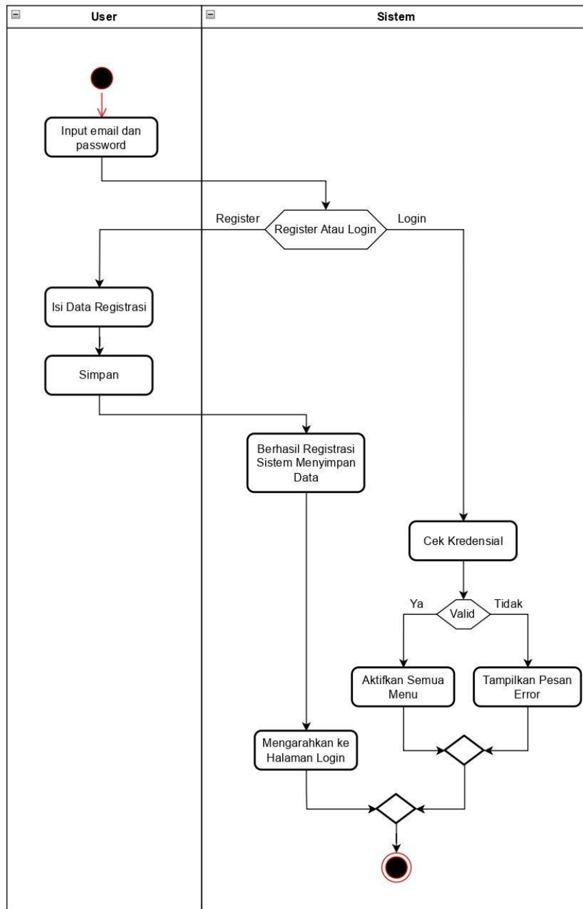
Gambar 3. 2 Login & Register Pengguna
