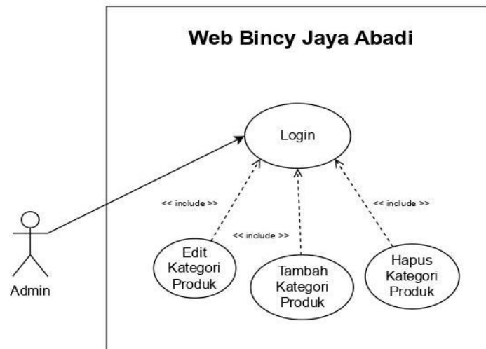
Gambar 3. 17 Use case Admin Kategori
